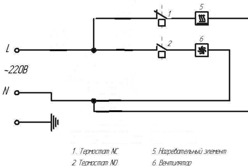
Схема электрическая принципиальная
