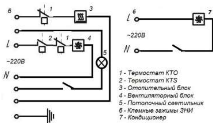
Рис. 5. Схема электрическая
