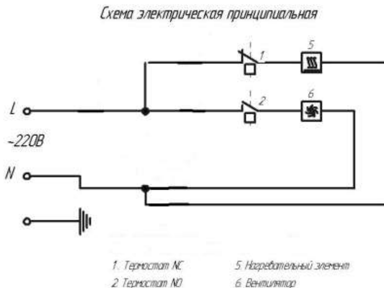
Рис. 5. Схема электрическая
