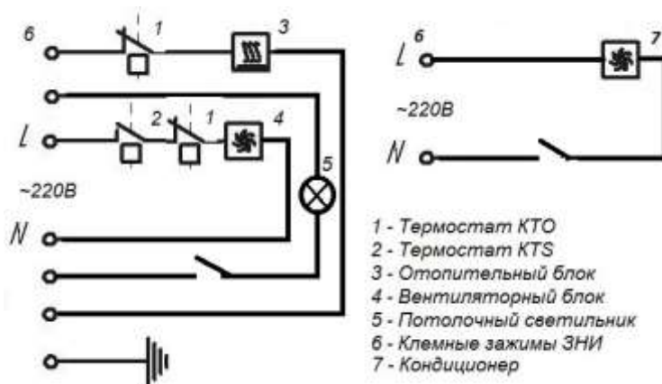
Рис. 5. Схема электрическая
