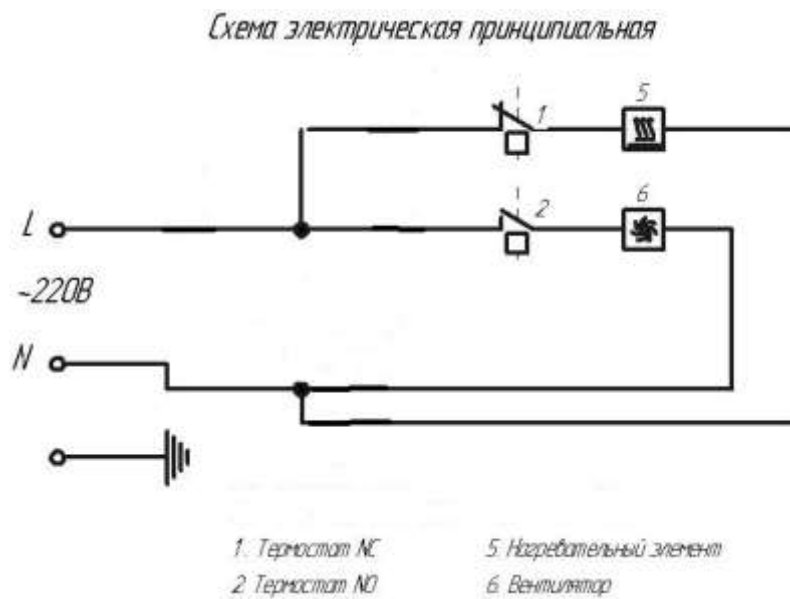
Рис. 5. Схема электрическая
